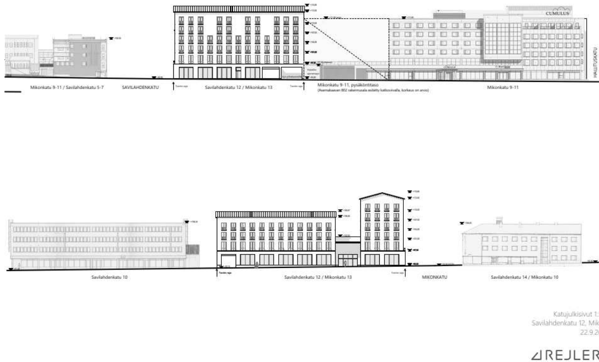
Kuva 16. Uudisrakennuksen katujulkisivut (Rejlers Rakentaminen Oy, 2026).
