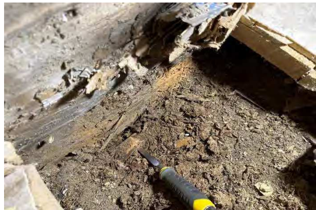
Kuva 63. Ulkoseinän alaosan lahovauriota.
