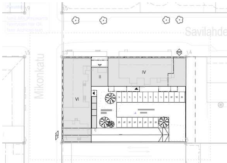
Kuva 14. Viitesuunnitelman asemapiirustus.
