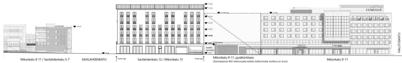
Kuva 17. Katuleikkaus Mikonkadulta (idän suunnasta). Kuvassa on esitetty naapurikiinteistön asemakaavan 802 käyttämätön rakennusala katkoviivalla, korkeus arvioitu.
